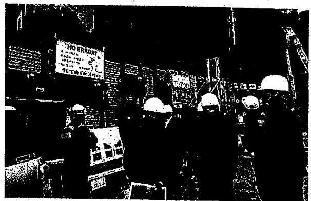
写真13 地すべり防止施設(深礎工)の視察 (B班)
