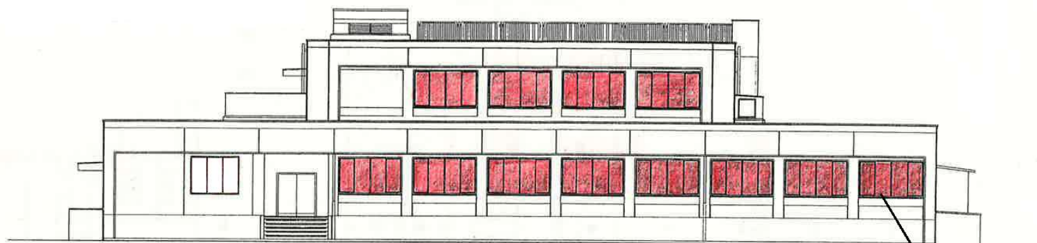
南 立 面 図
