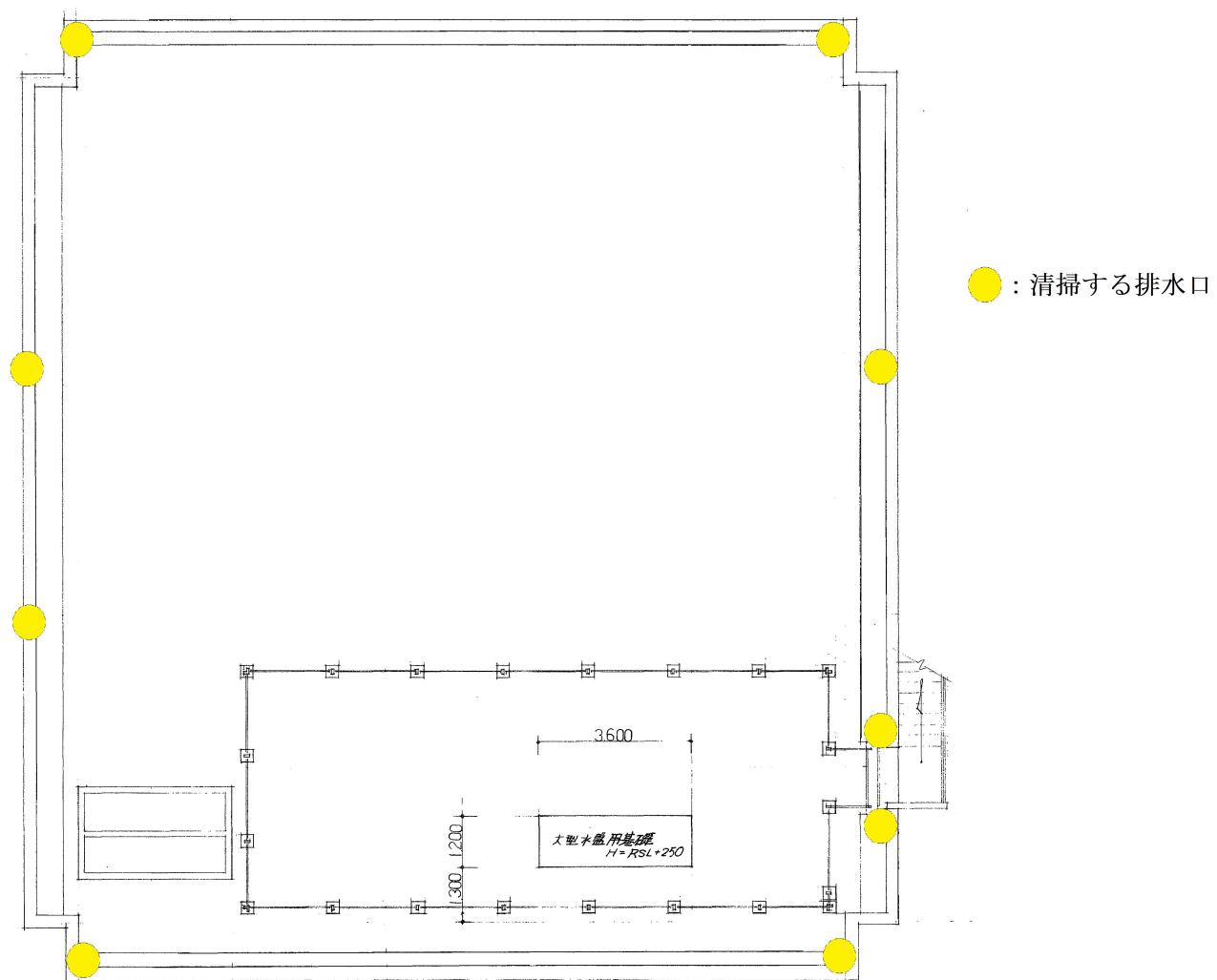
R 階 平 面 図
