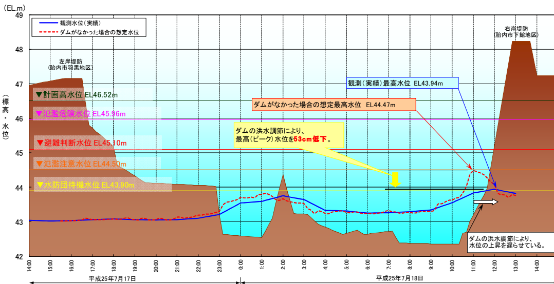
胎内川 下館観測所地点の水位状況図 -ダムの貯水による効果-
