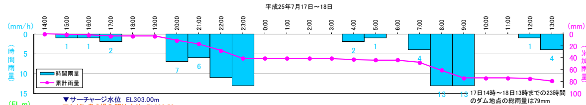
胎内川ダム ダム操作状況図 -ダムの動き-
