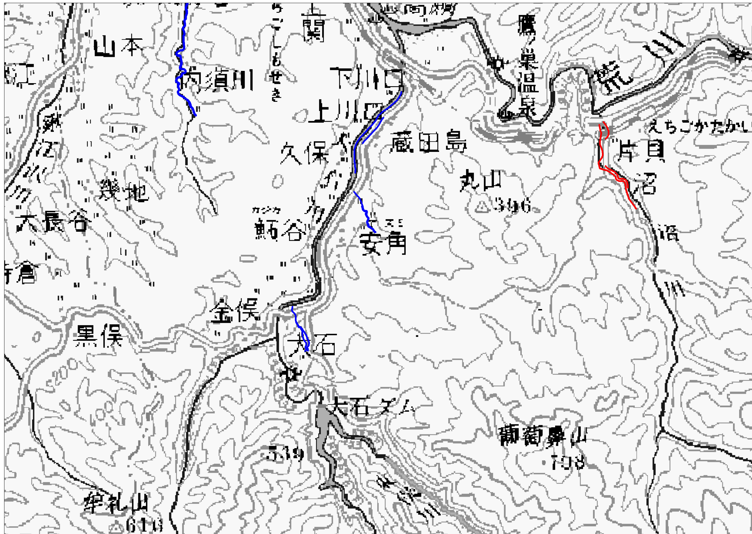
改修実績に基づく治水安全度評価（拡大図 3）
