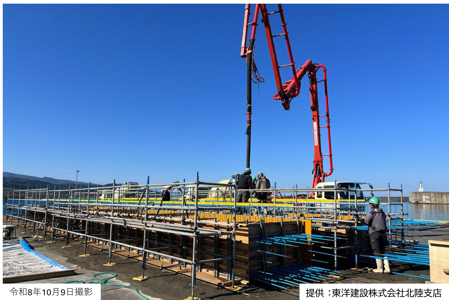
製作状況（コンクリート打設）
