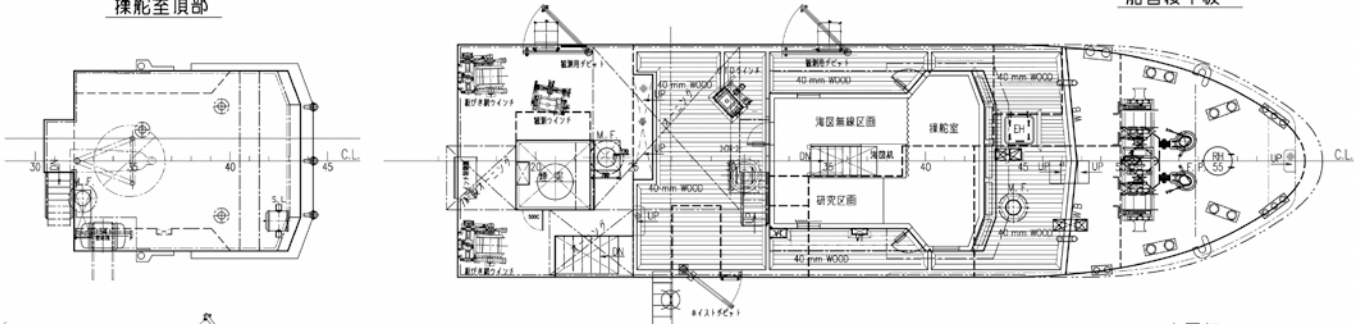
上甲板
