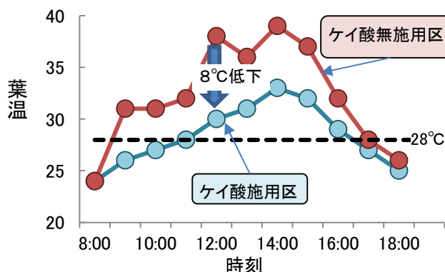
図1 高温条件における葉温に及ぼすケイ酸の効果 参照:「金田ら、ケイ酸質肥料が高温処理水稻の葉温・気孔コンダクタンス・ケイ酸吸収に及ぼす影響、日本土壌肥料科学雑誌第81巻、2010」
