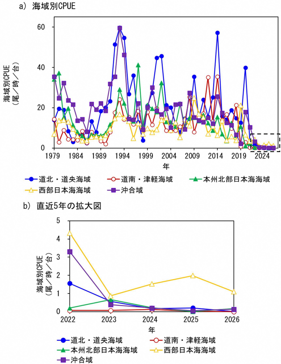
図3. 日本海におけるいか釣り調査による海域別CPUEの年推移 直近5年（上図aの破線で囲まれた年）を拡大したものを下図bで示した。
