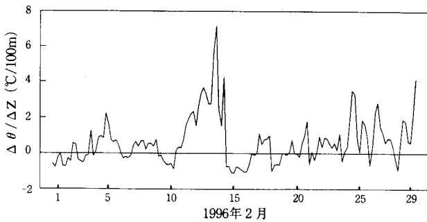
図8 1996年2月の温位傾度の変化 (東新潟火力発電所)
