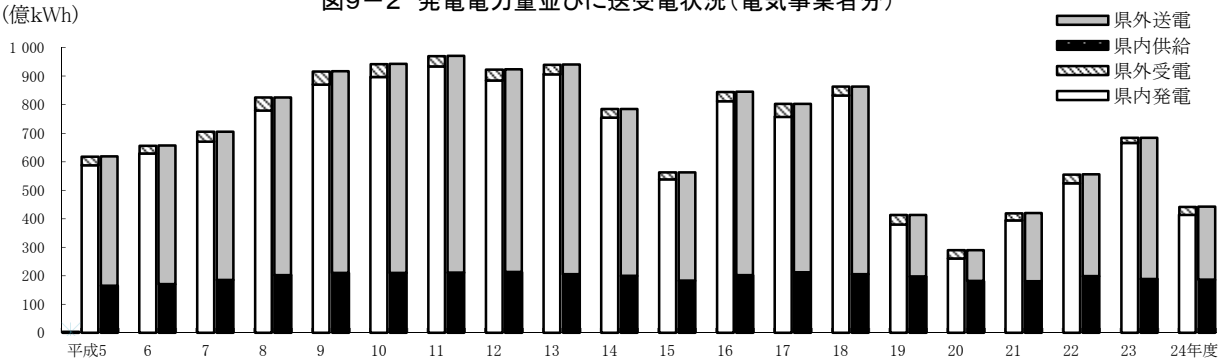
図9-2 発電電力量並びに送受電状況(電気事業者分)
