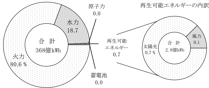
図9-2 発電電力量の構成(令和5年度)
