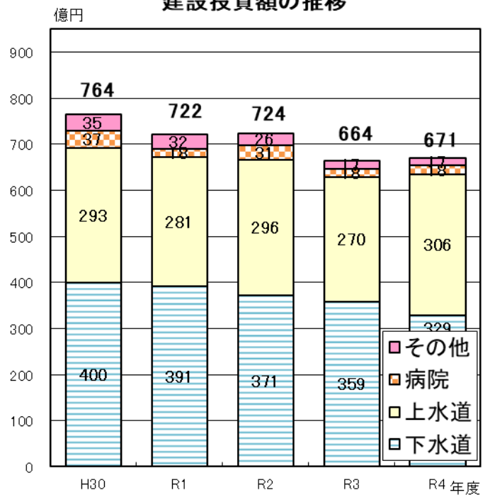
建設投資額の推移
