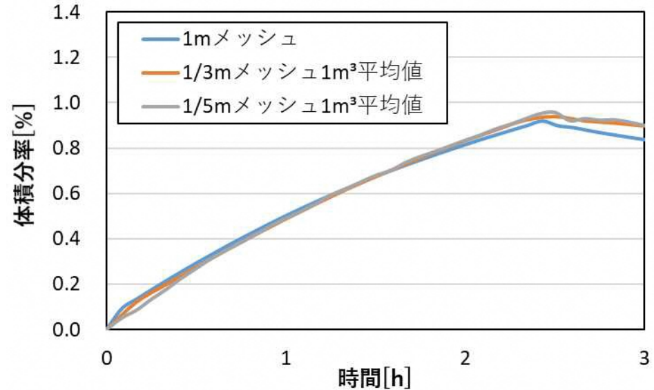
各解析の体積1m 3 における水素濃度比較
