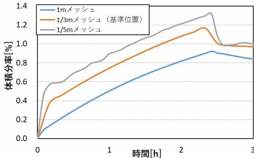
各解析の1メッシュでの水素濃度比較
