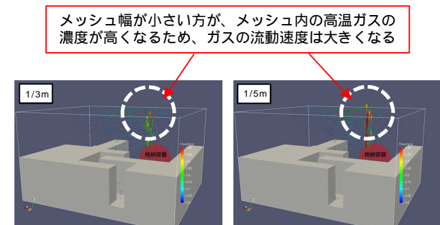
初期過渡領域 (4)(5) ガス流動の速度ベクトル
