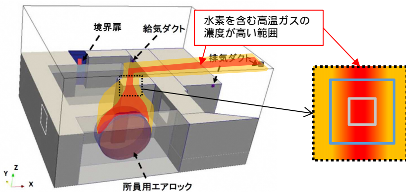
事象初期の水素を含む高温ガス濃度分布イメージ
