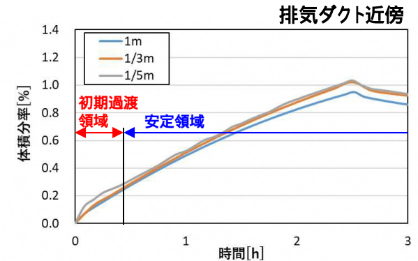
排気ダクトにおけるメッシュ幅毎の水素濃度時刻歴
