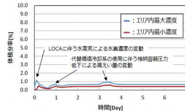
下部ドライウエル所員用エアロック室における水素濃度の時間変化
