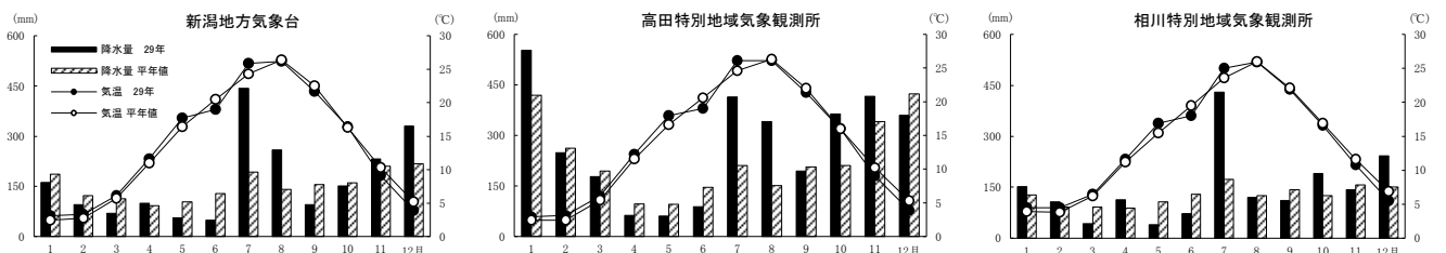
図1-2 気温と降水量 (平成29年と平年値)
