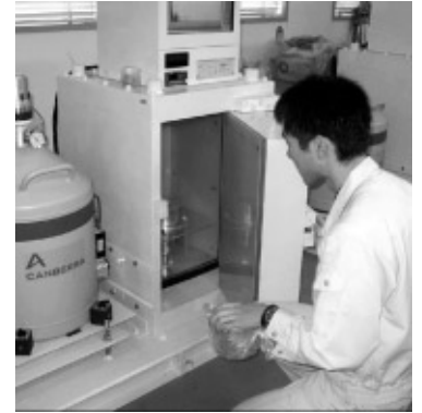
ゲルマニウム半導体検出器
