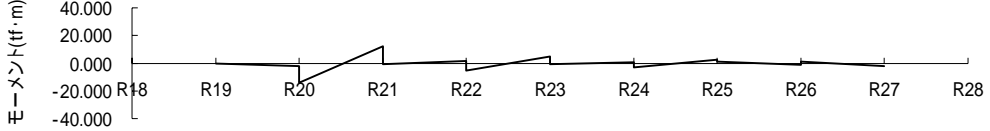
c. 曲げモーメント(床版)
