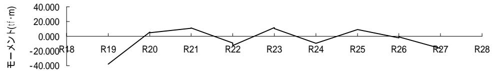
c. 曲げモーメント(床版)
