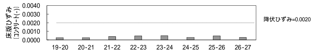
h. 床版ひずみ(コンクリート)
