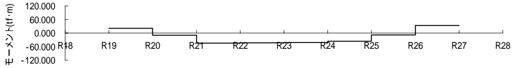
b. 曲げモーメント(上弦材)
