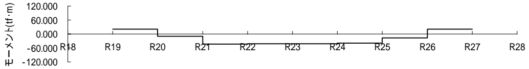
b. 曲げモーメント(上弦材)
