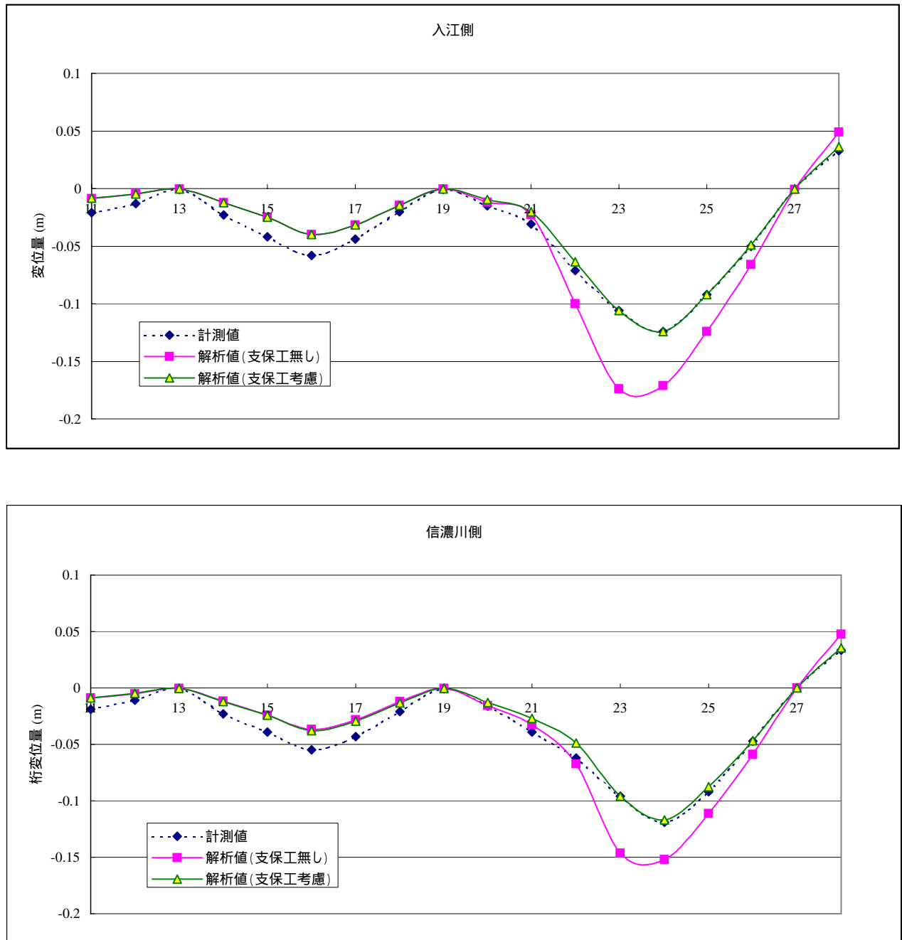
図 2 最初のジャッキダウン時のたわみ状態
