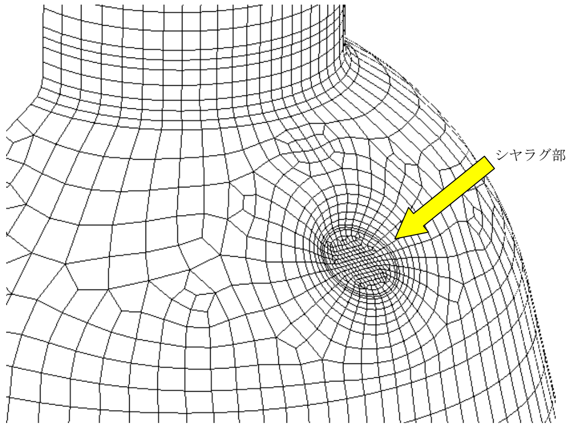
内側メイルシヤラグに鉛直方向荷重が作用した場合の 原子炉格納容器胴の変形図（変形倍率：3000倍）
