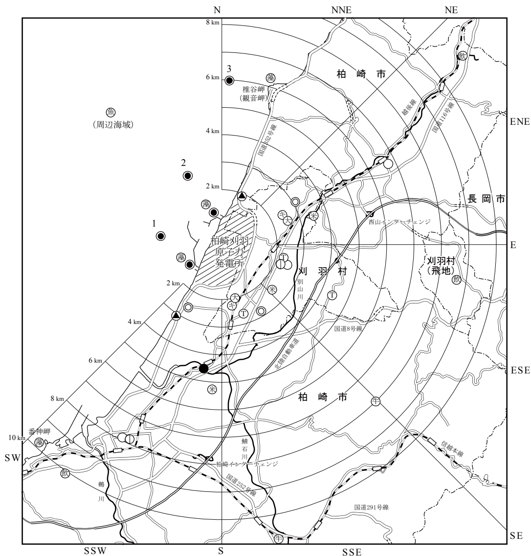
図-2 環境試料採取地点
